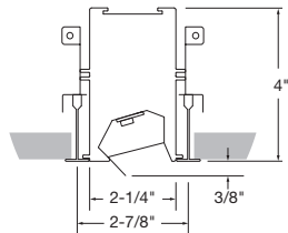
9/16" T-Bar (C2)
