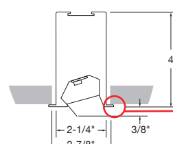
Visible Flange (VF)
