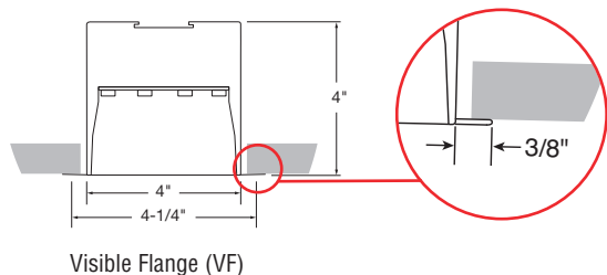
Visible Flange (VF)
