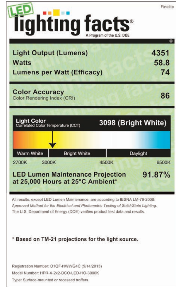
HPR-LED 2x2 DCO HO 3000K
