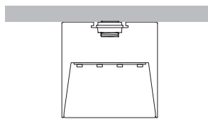
HP-4 WL SM 3
