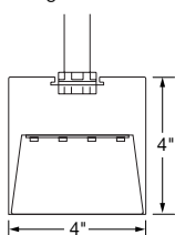
Pendant Rigid Stem
